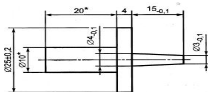
Рисунок 1 — Испытательный палец
