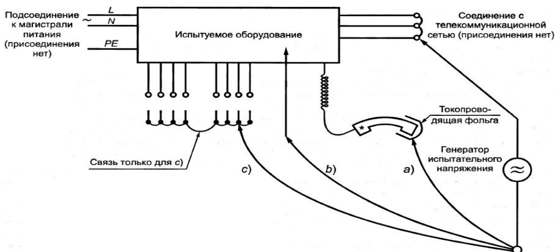
Рисунок 18 – Точки приложения испытательного напряжения
