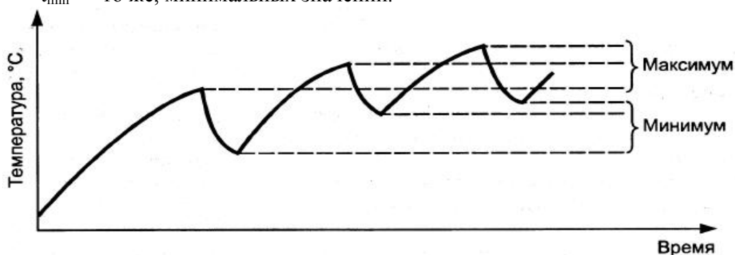
Рисунок Б. 1 – Определение среднеарифметической температуры
