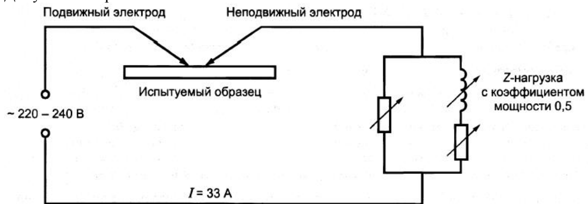
Рисунок А.1 – Схема испытания на возгораемость от сильноточного дугового разряда
