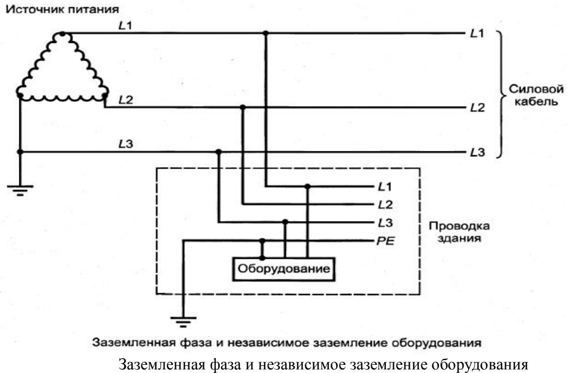
Рисунок Ф.6- Пример трехпроводной ТТ системы энергоснабжения
