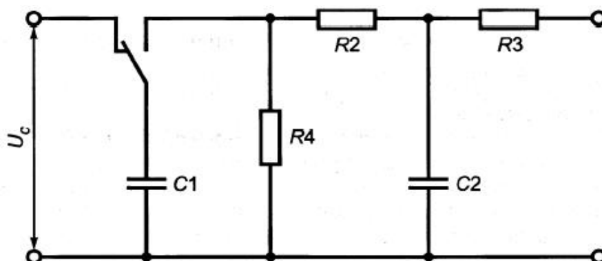
Рисунок П.1 – Схема генератора импульсов
