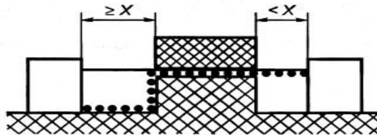
Рисунок Е.6 – Несплошной стык с широкими канавками
