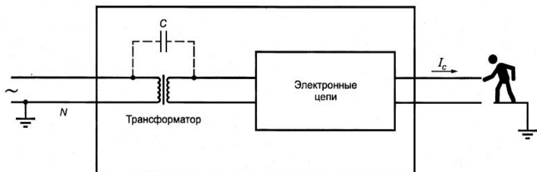
Рисунок X.1 – Прикосновение к изменяющейся цепи
