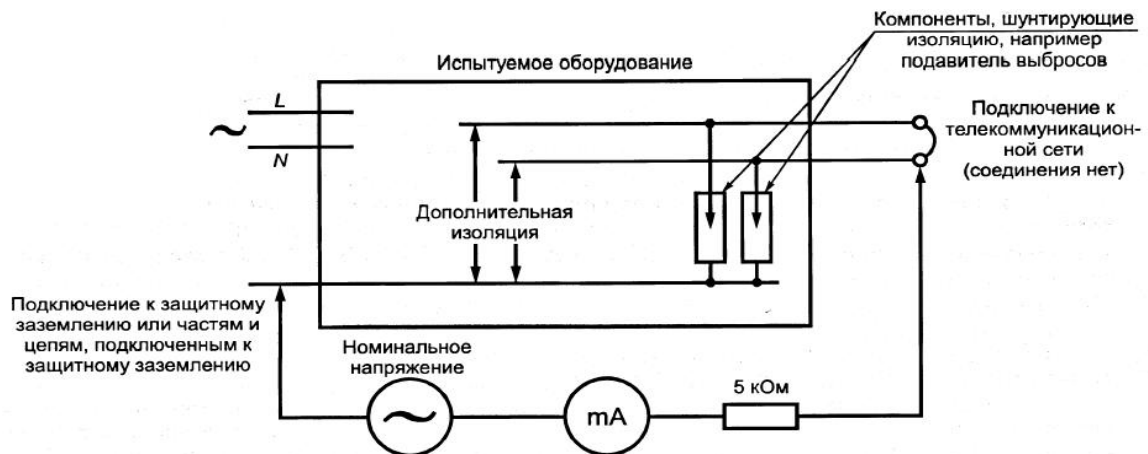
Рисунок 17 – Испытание развязки между телекоммуникационной сетью и «землей»
