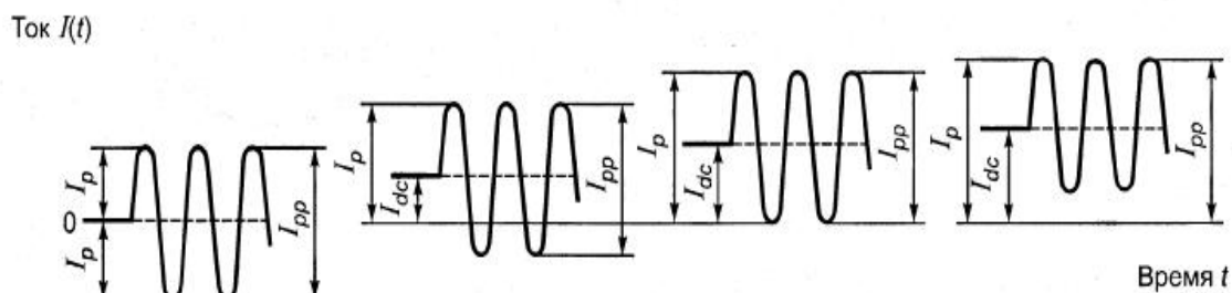
Рисунок Н. 3 – Амплитуда и размах амплитуд тока
