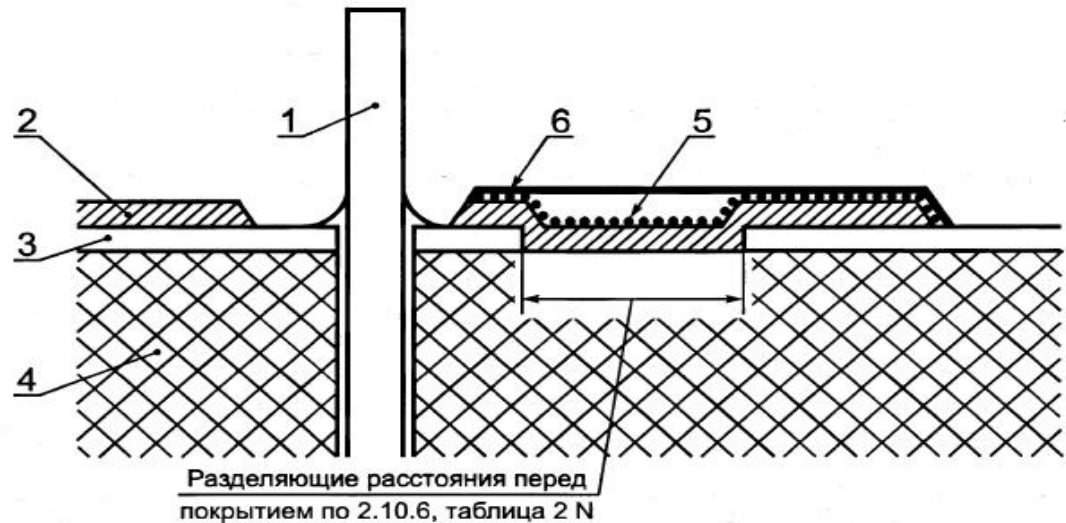
Рисунок Е. 11 – Покрытие поверх печатных проводников
