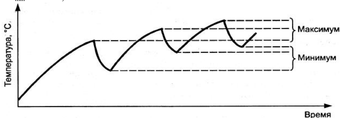
Рисунок В.1 — Определение среднеарифметической температуры
