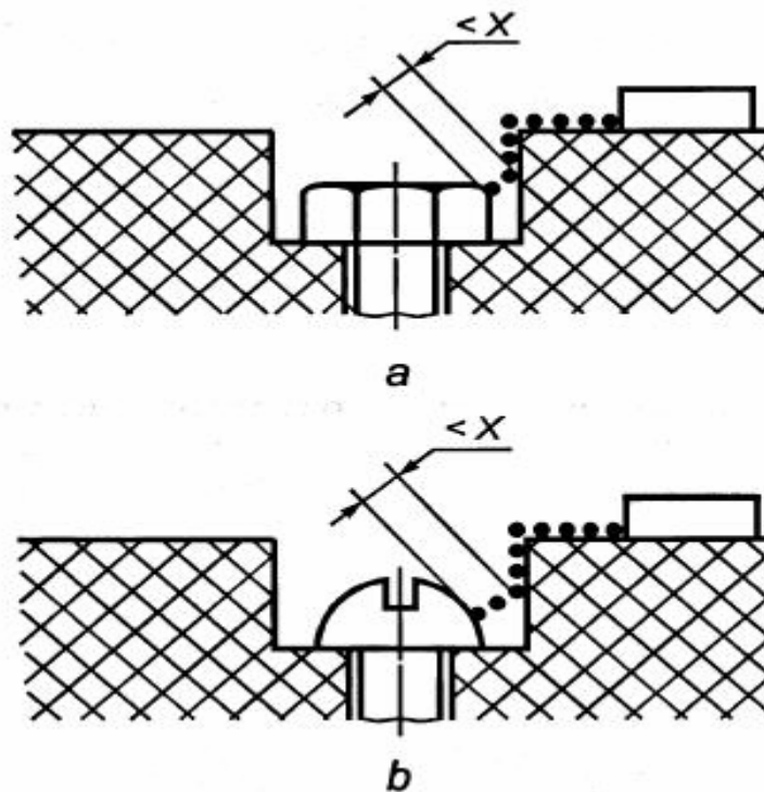
Рисунок Е.7 – Несплошной стык с узкой и широкой канавками
