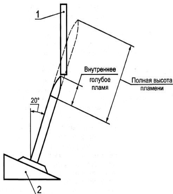
Рисунок А.4 – Установка для испытания вертикальным пламенем материала каласса
