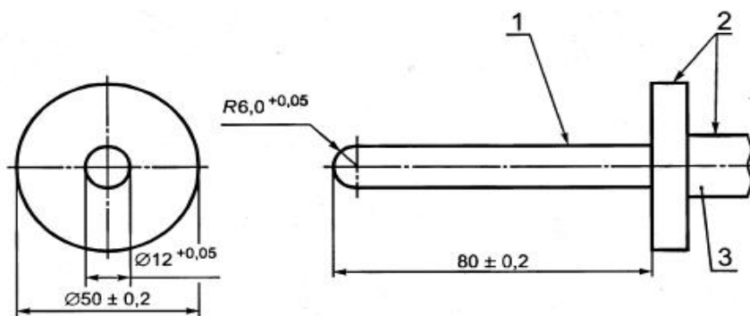
Рисунок 3 – Испытательный калибр
