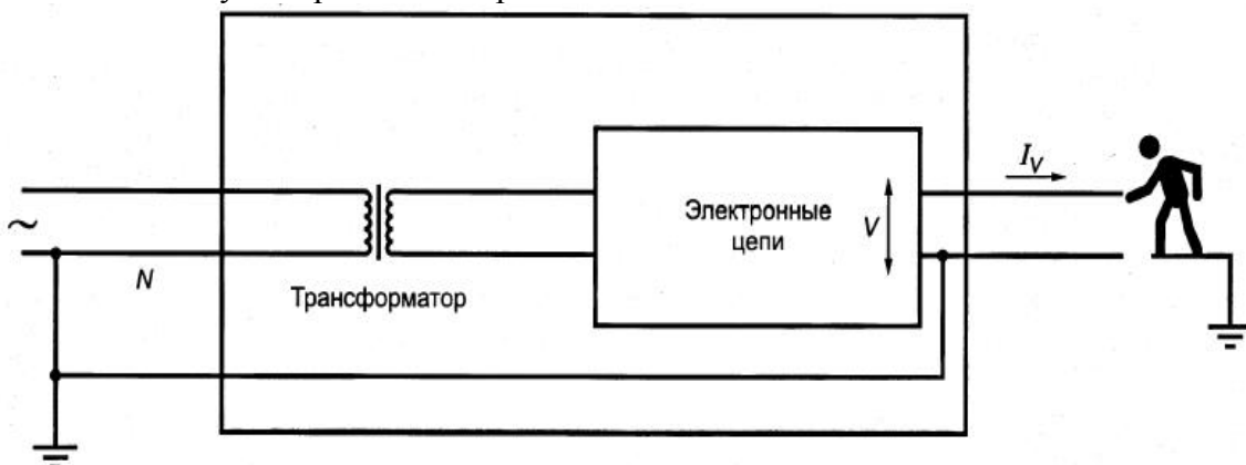
Рисунок X.2 – Ток прикосновения от заземленной цепи
