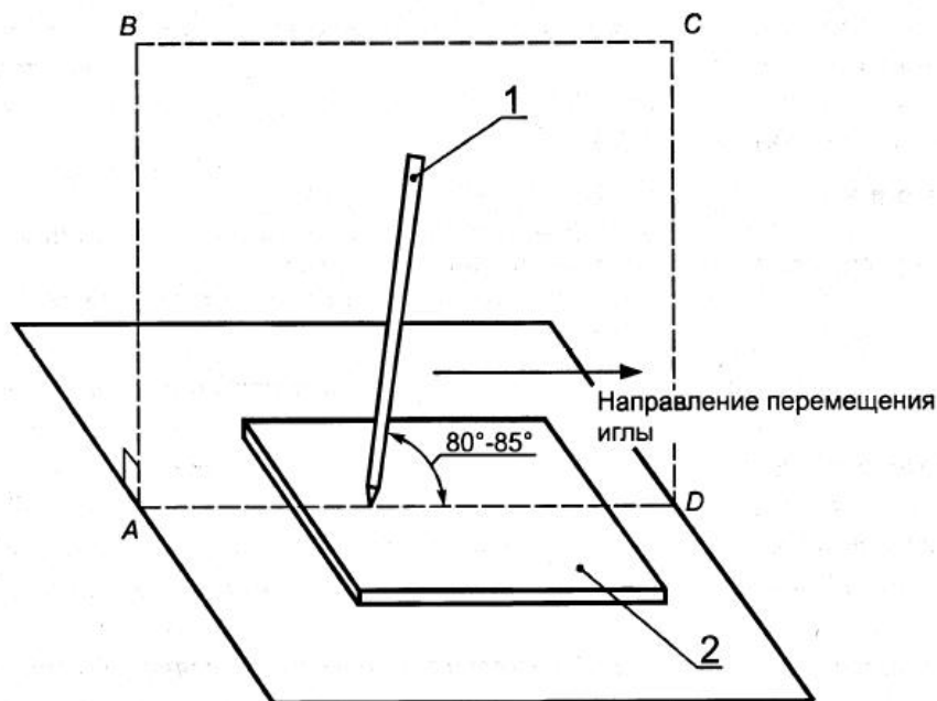
Рисунок 8 – Испытание покрывающего слоя на износостойкость
