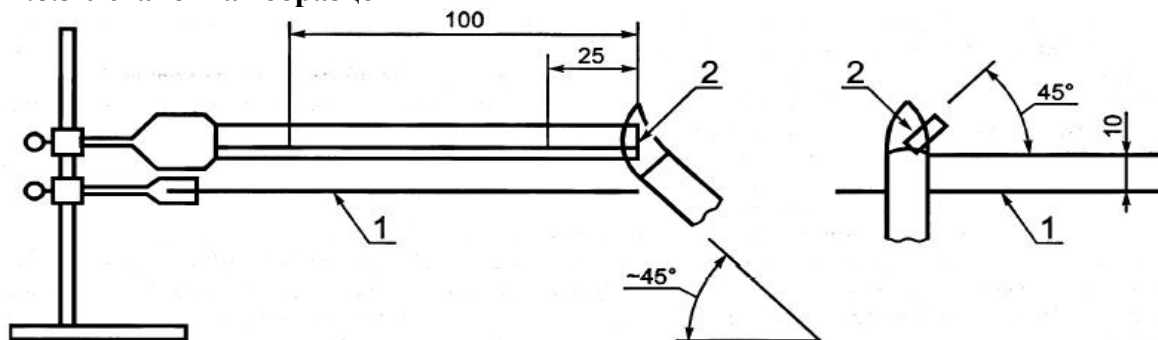
1 — сетка; 2 — испытываемый образец
