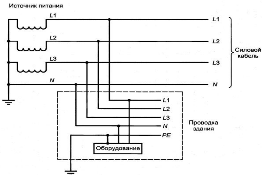
Рисунок Ф.5 – Пример трехфазной линии и нейтрали ТТ системы энергопитания
