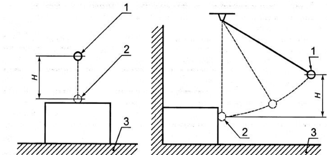
1 — начальное положение шара; 2 — положение шара в момент удара; 3 — твердая поверхность Условия соответствия по — 6.2.1.
