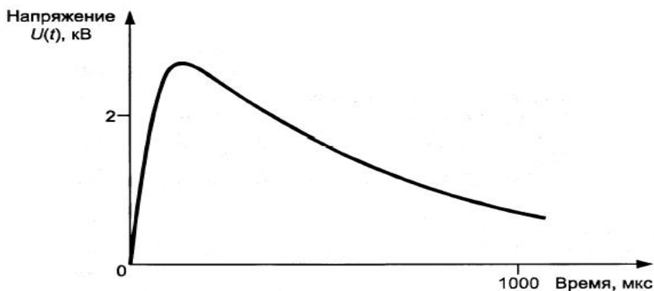
Рисунок С.1-Форма сигнала при испытании изоляции (ограничитель выбросов отсутствует, пробой изоляции нет)
