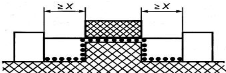
Рисунок Е.5 – Несплошной стык с узкими канавками
