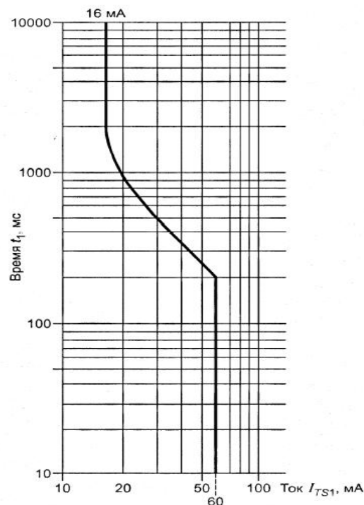
Рисунок Н. 2 – Кривая предельного значения тока I_{TS1} модулированного сигнала звонка
