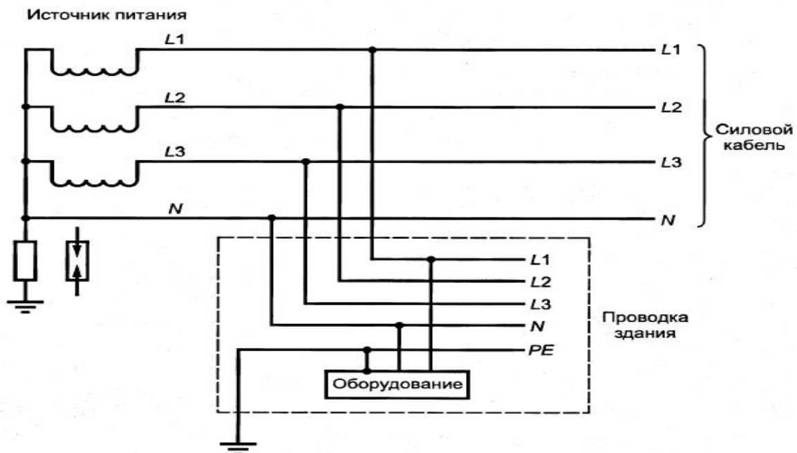
Рисунок Ф.7 – Пример трехпроводной (с нейтралью) IT системы энергоснабжения.
