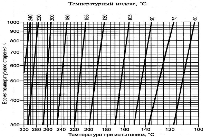
Рисунок 7 – Время теплового старения
