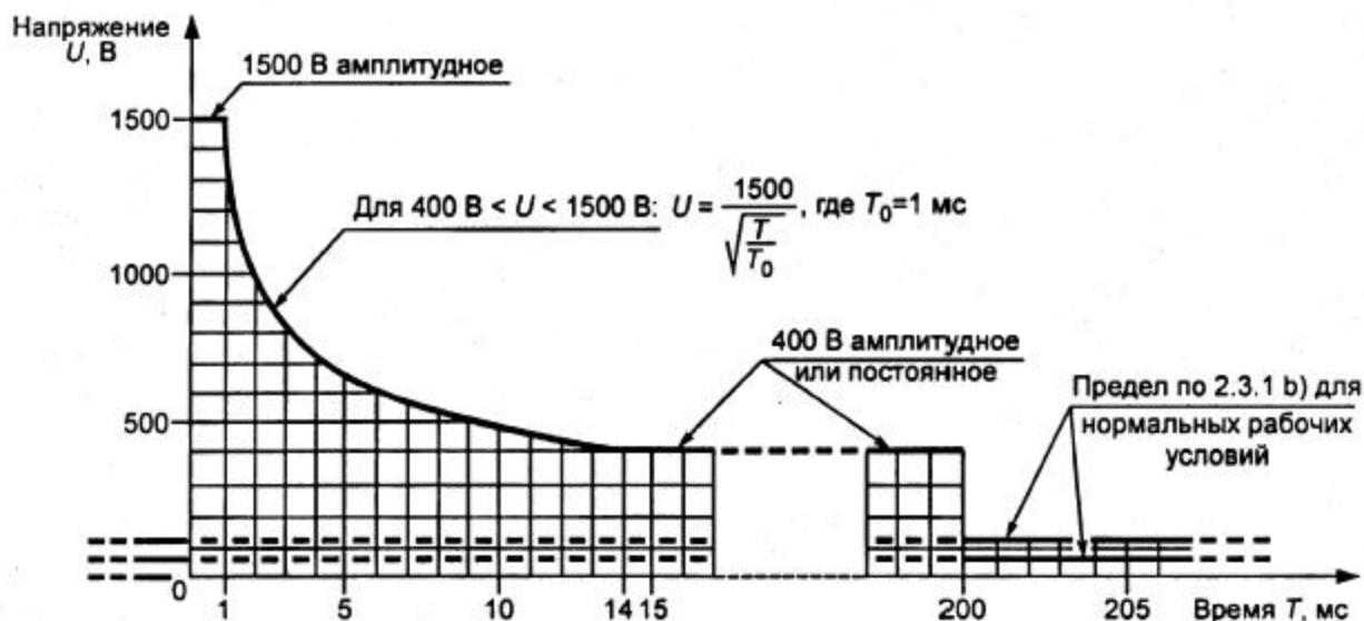
Рисунок 4 — Максимальное напряжение, допускаемое после единичного повреждения изоляции
