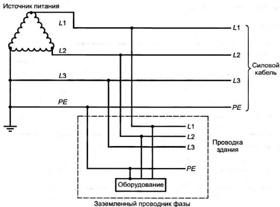
Рисунок Ф.1 – Пример TN-S системы энергоснабжения
